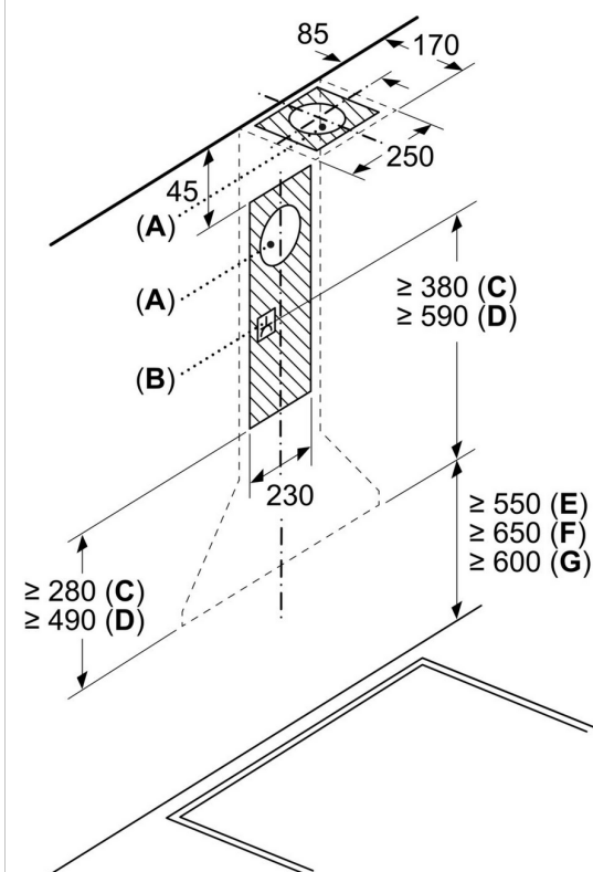
Dimensiones en mm
