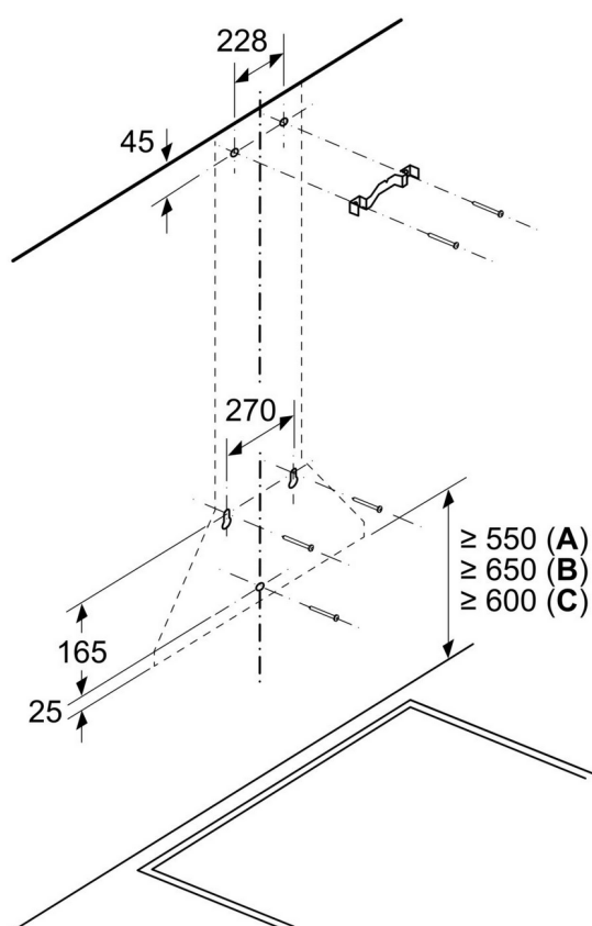
Dimensiones en mm
